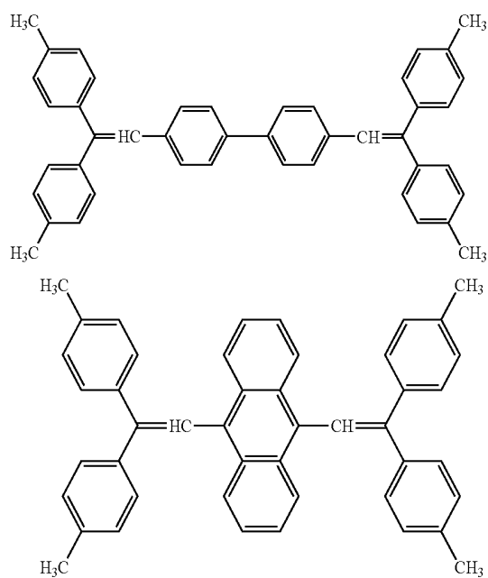
BCP
